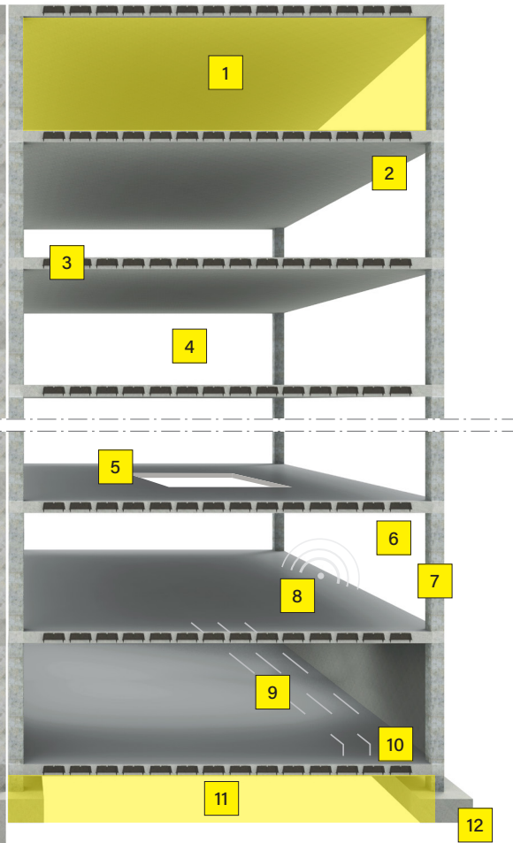
SISTEM OPTIMIZAT CU SISTEMUL U-BOAT BETON
